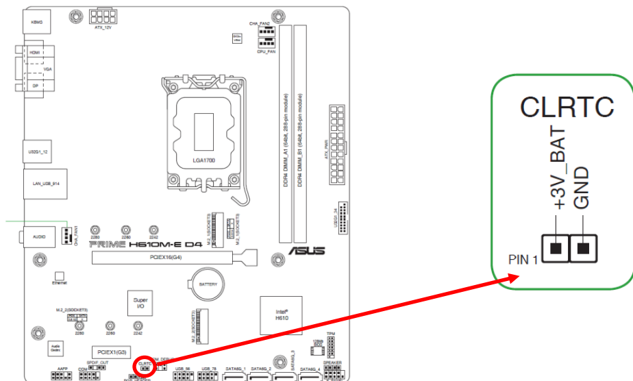
Figure 4.15 Emplacement du bloc de cavalier de configuration du BIOS
