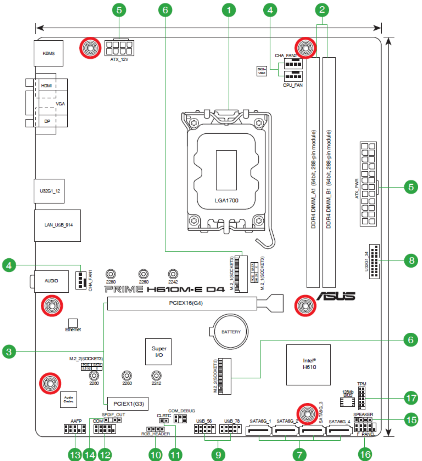
Schéma 4.4 Composantes de la carte mère
