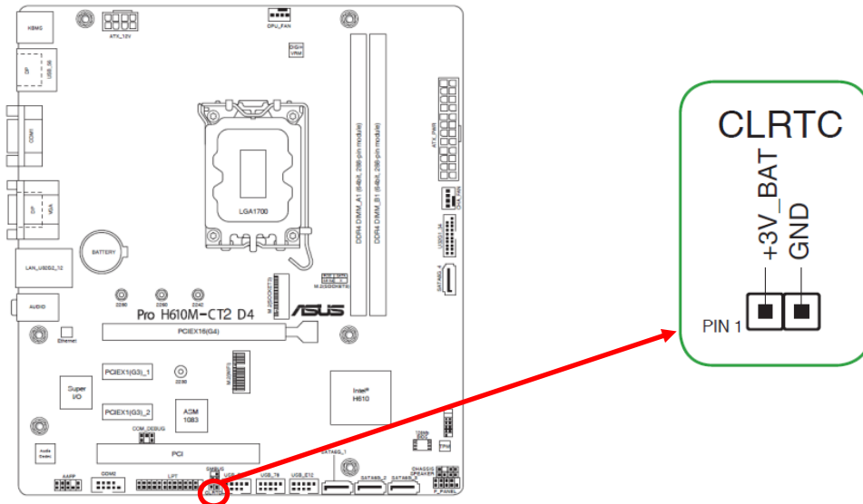
Figure 4.15 Emplacement du bloc de cavalier de configuration du BIOS
