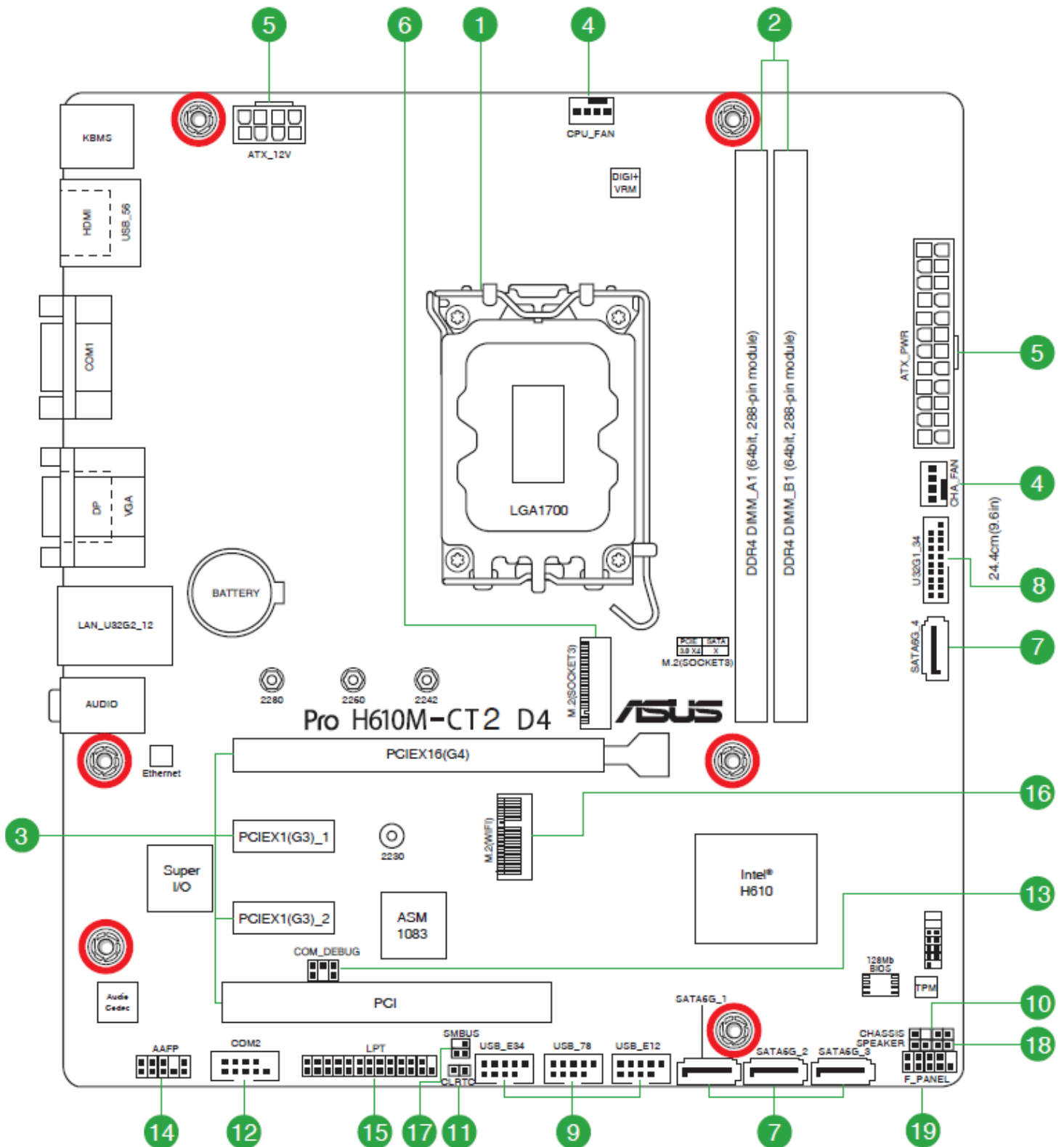
Schéma 4.4 Composantes de la carte mère
