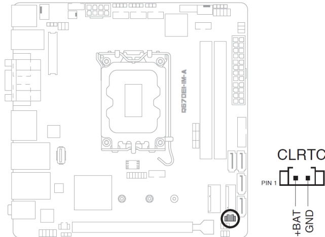
Figure 4.17 Emplacement du bloc de cavalier de configuration du BIOS
