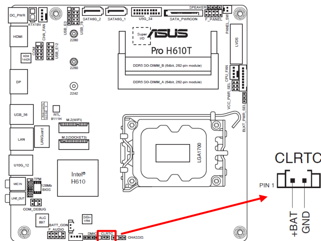
Emplacement du bloc de cavaliers de configuration du BIOS
