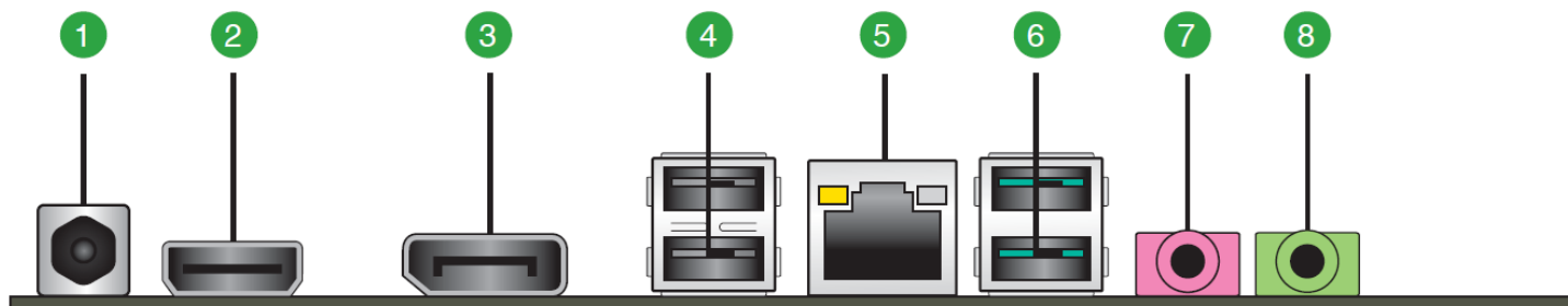
Schéma 4.5 Connecteurs du tableau arrière
