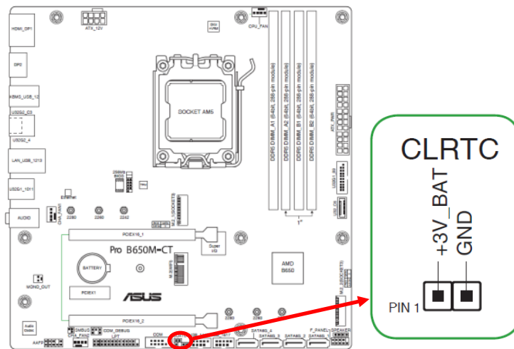
Figure 4.17 Emplacement du bloc de cavalier de configuration du BIOS
