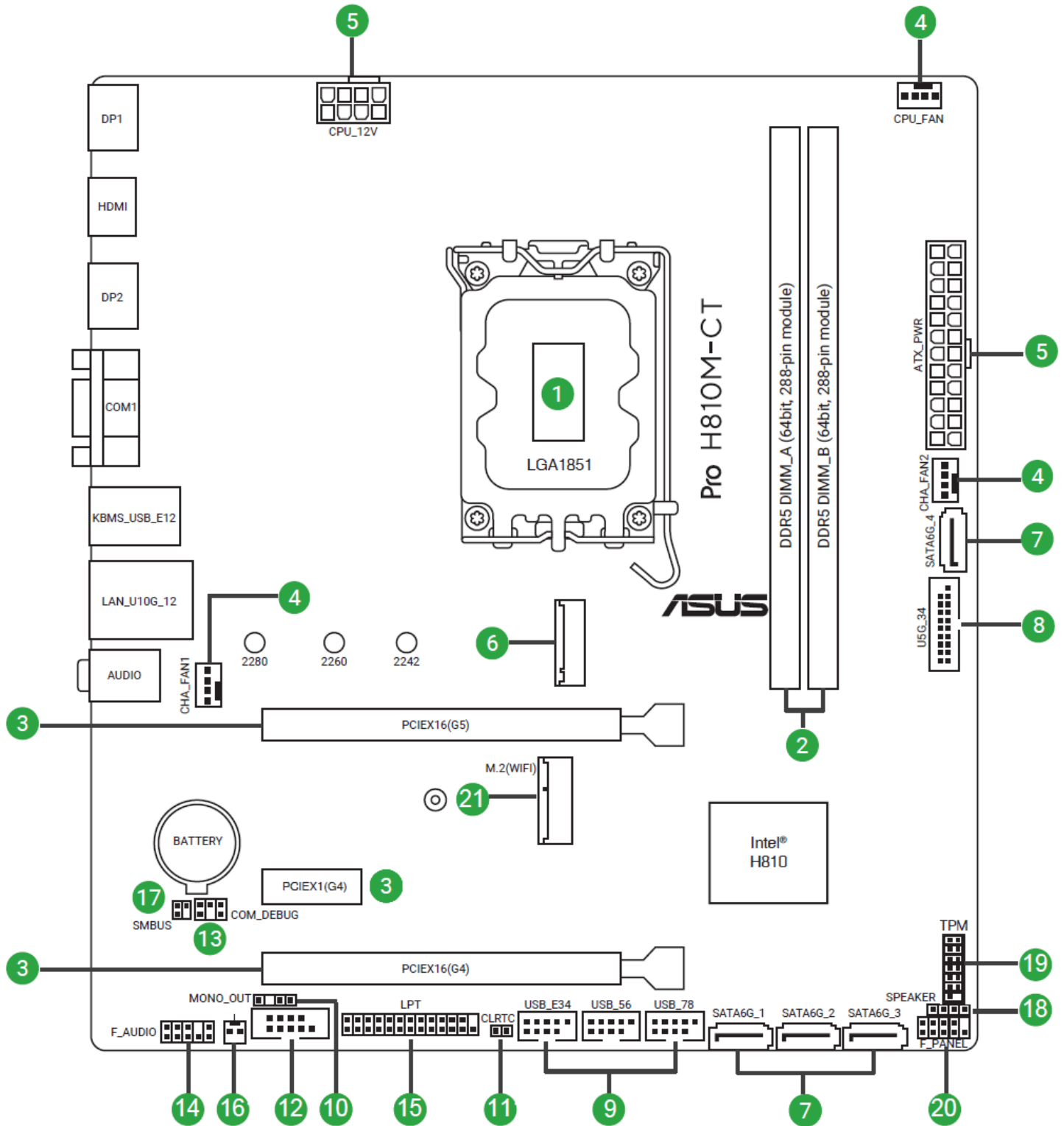
Schéma 4.4 Composantes de la carte mère
