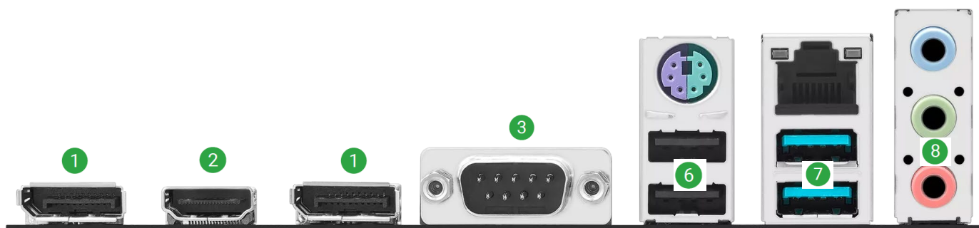
Schéma 4.5 Connecteurs du tableau arrière
