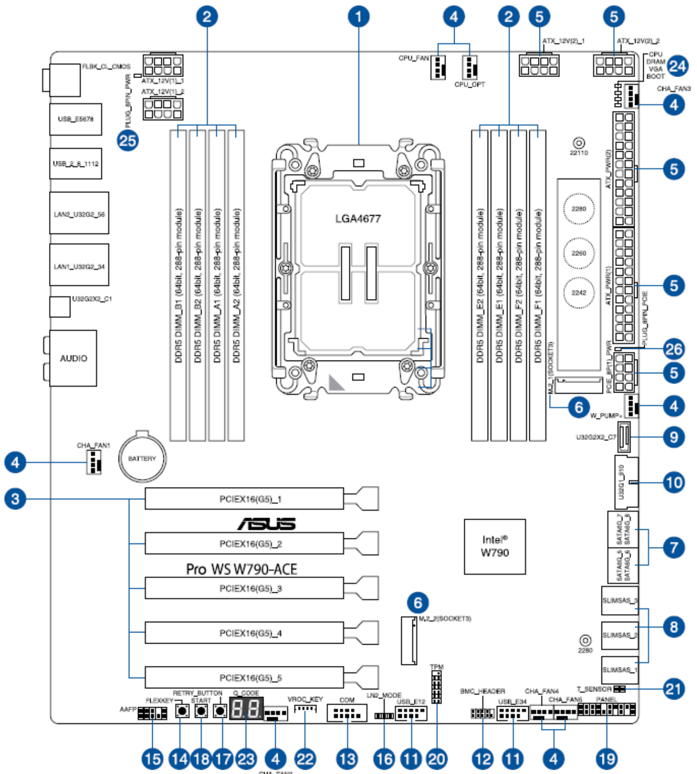
Schéma 4.4 Composantes de la carte mère
