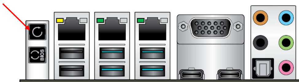
Figure 4.16 Emplacement du bouton de réinitialisation du CMOS
