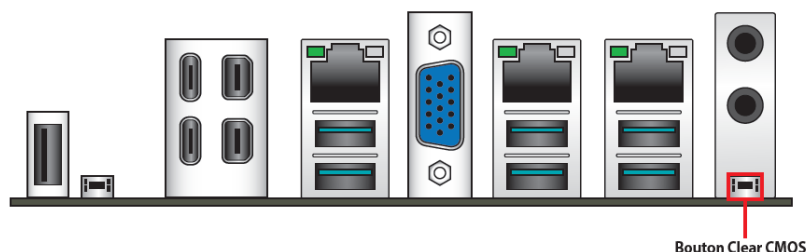
Figure 4.16 Emplacement du bouton de réinitialisation du CMOS
