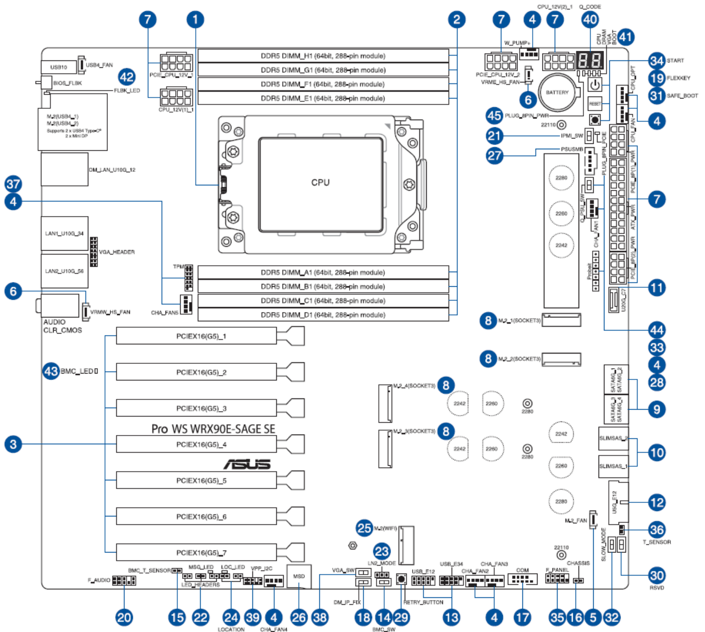
Schéma 4.4 Composantes de la carte mère
